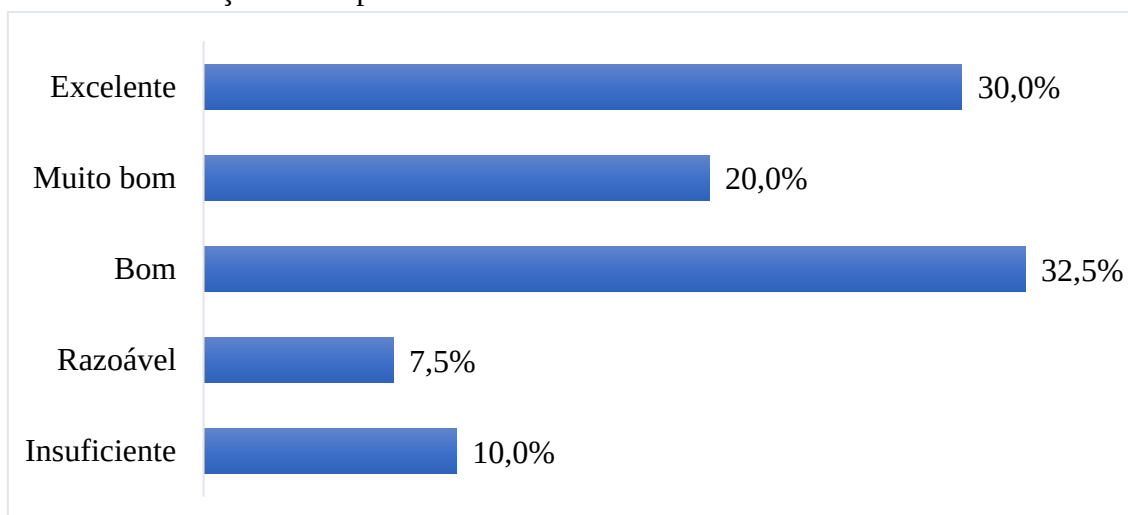
Gráfico 8 – Relação teoria-prática.
